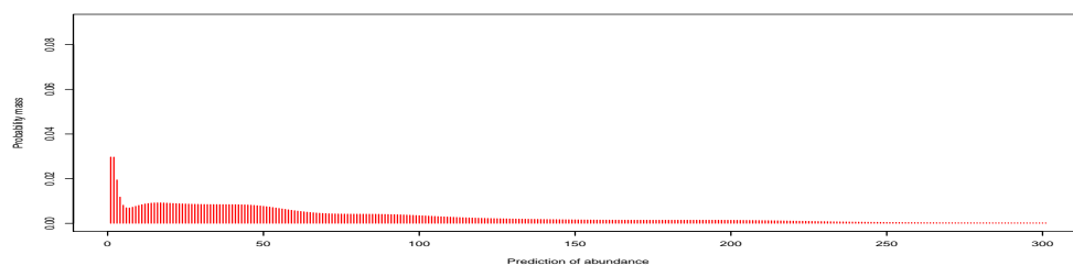
(d) \sigma = 0.75
