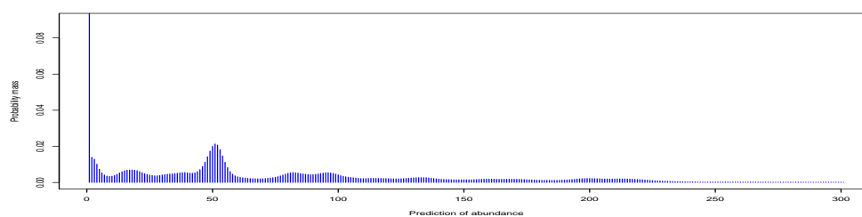
(d) \sigma = 0.75
