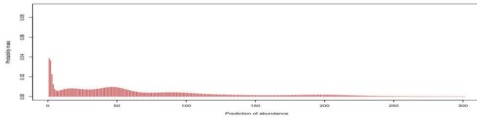
(d) \sigma = 0.75
